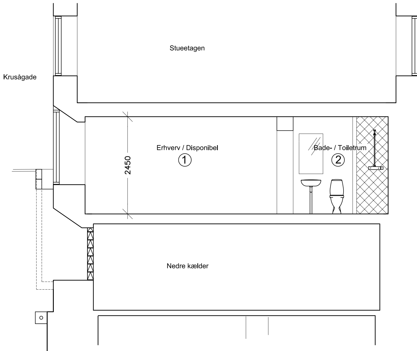
TVÆRSNIT A-A. MÅL 1:50.
