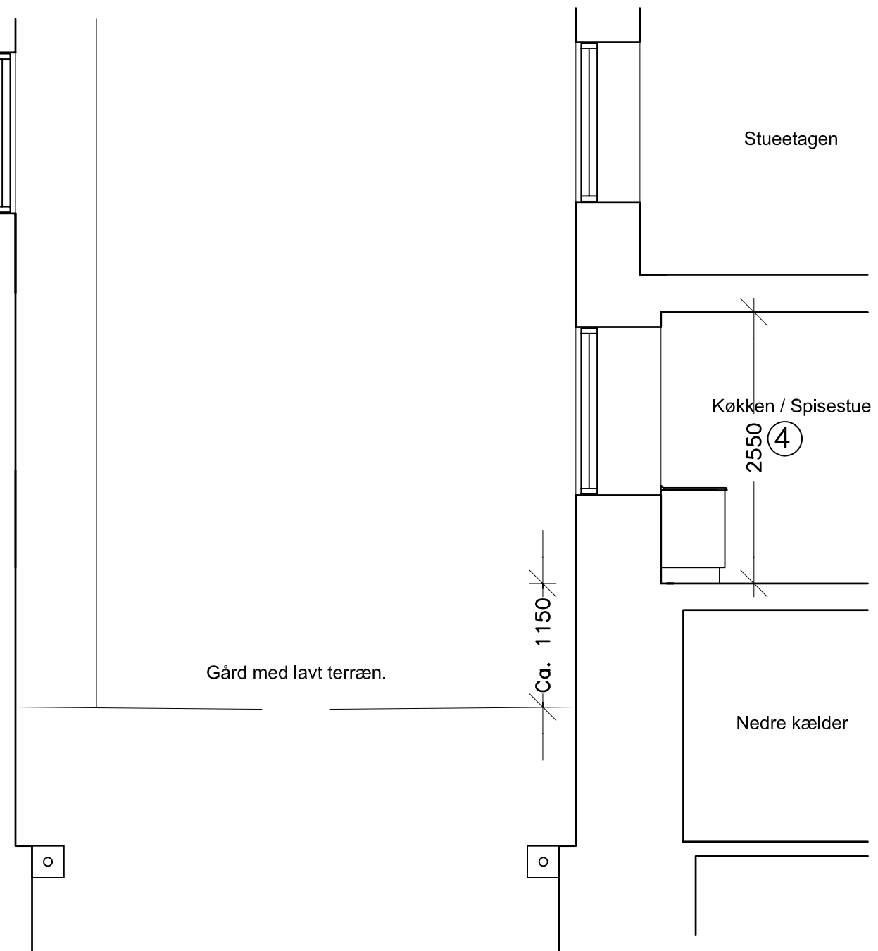
DELSNIT B. MÅL 1:50.
